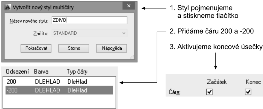
Obrázek č. 3.44: Nastavení stylu multičáry pro kreslení obvodového zdiva
