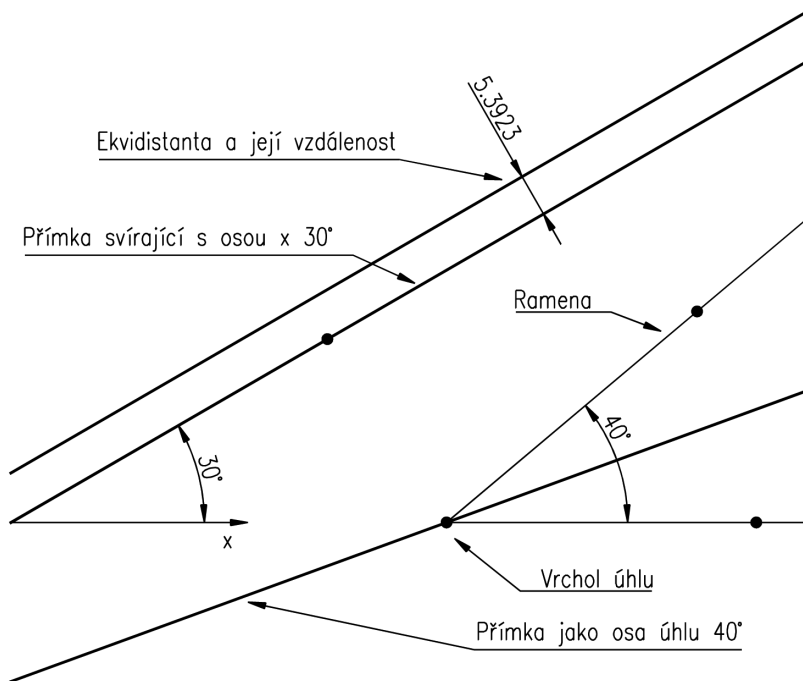
Obrázek č. 3.27: Parametry konstrukčních čar
