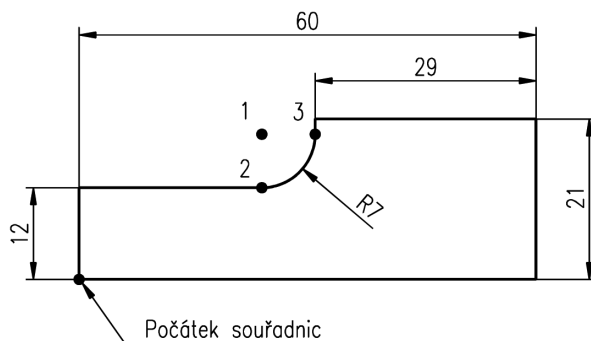
Obrázek č. 3.15: Konstrukce oblouku
