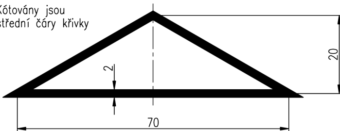
Obrázek č. 3.32: Konstrukce křivky s definovanou tloušťkou
