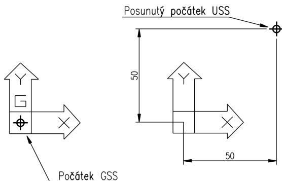
Obrázek č. 2.17: Posun počátku souřadného systému
