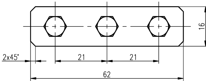
Obrázek č. 3.13: Kreslení polygonu – cvičení
