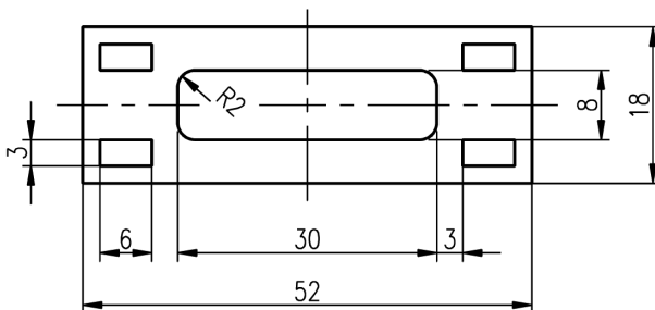
Obrázek č. 3.11: Kreslení obdélníku – cvičení
