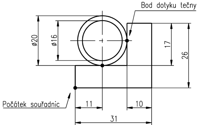
Obrázek č. 3.7: Konstrukce kružnice pomocí tečen
