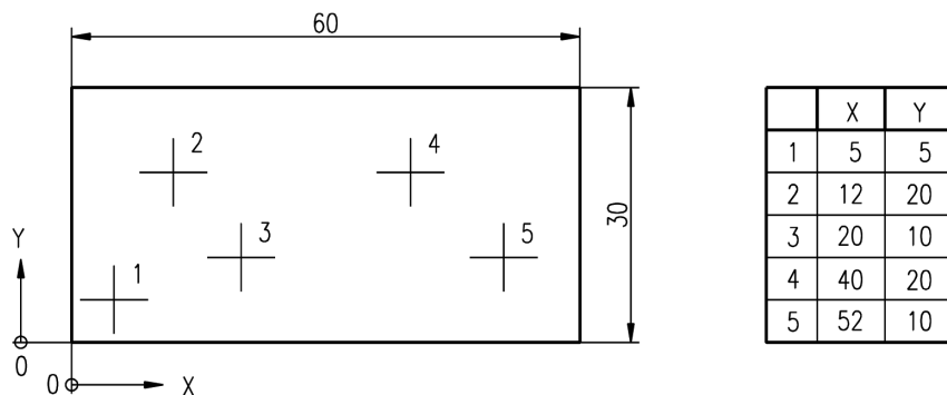
Obrázek č. 3.25: Kreslení bodů – cvičení
