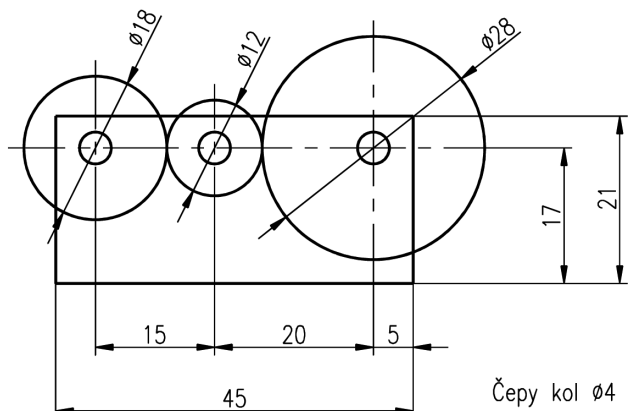
Obrázek č. 3.9: Kreslení kružnice – cvičení
