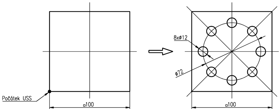
Obrázek č. 3.8: Kreslení děr na roztečné kružnici – cvičení
