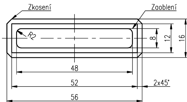
Obrázek č. 3.10: Možnosti konstrukce obdélníku
