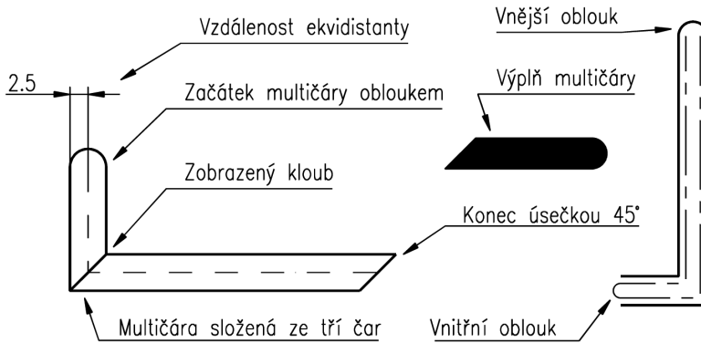
Obrázek č. 3.42: Parametry multičáry
