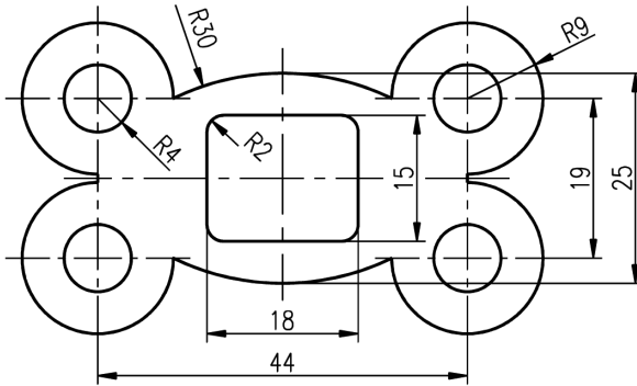
Obrázek č. 3.16: Kreslení oblouku – cvičení
