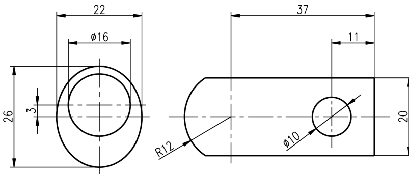
Obrázek č. 3.21: Kreslení elipsy – cvičení
