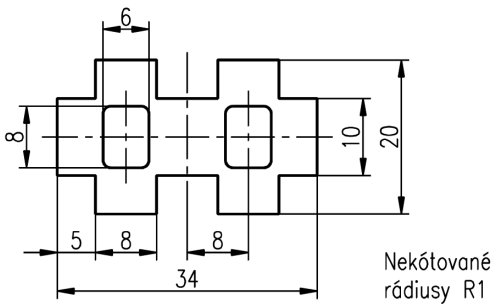
Obrázek č. 3.41: Kreslení křivek – cvičení
