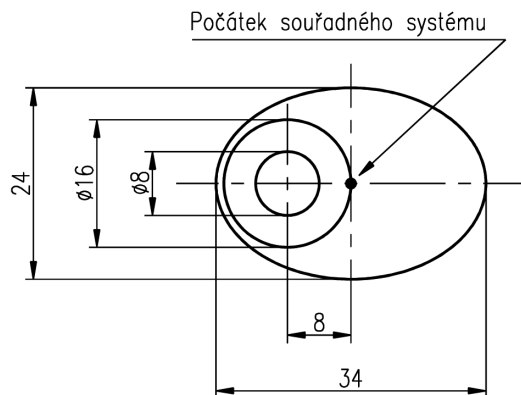
Obrázek č. 3.18: Konstrukce elipsy
