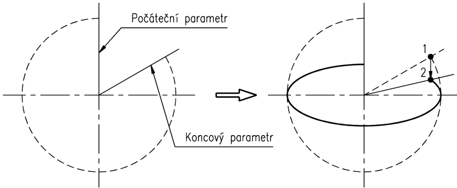
Obrázek č. 3.20: Konstrukce eliptického oblouku pomocí parametrů
