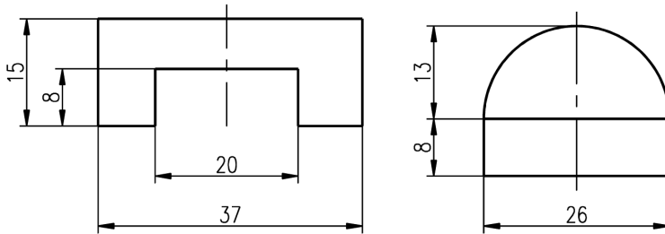
Obrázek č. 3.38: Kreslení křivek – cvičení
