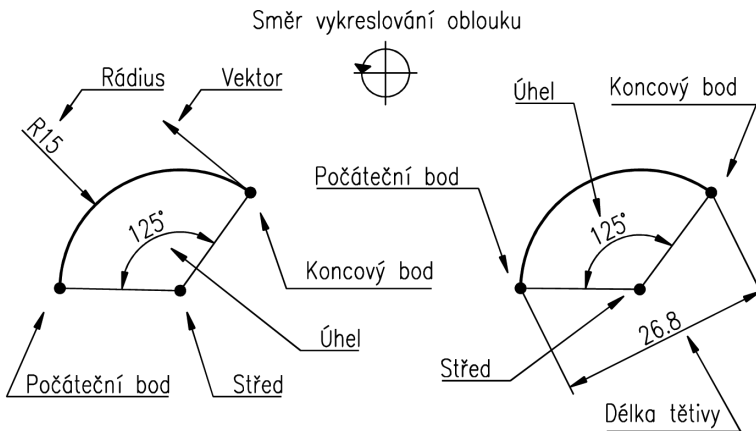
Obrázek č. 3.14: Parametry oblouku
