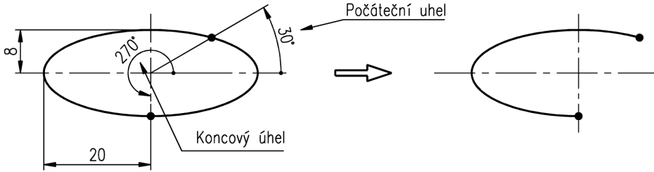
Obrázek č. 3.19: Konstrukce eliptického oblouku
