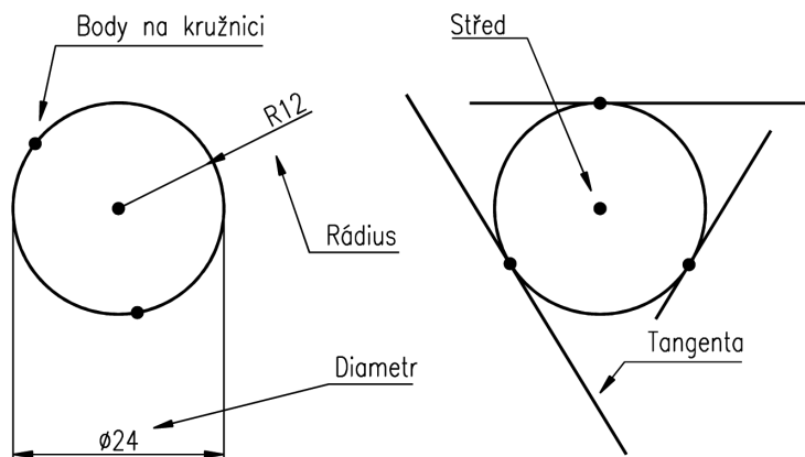
Obrázek č. 3.6: Parametry kružnice
