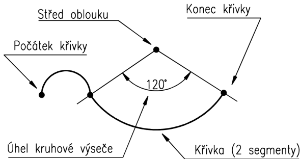
Obrázek č. 3.31: Parametry obloukových segmentů křivky
