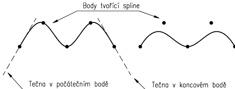
Obrázek č. 3.39: Konstrukce spline křivky
