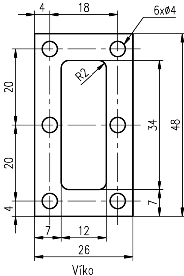
Obrázek č. 3.28: Konstrukční přímky – cvičení
