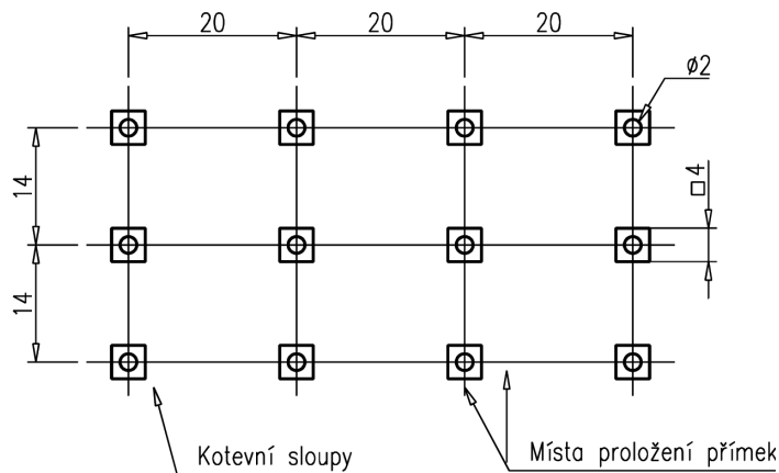
Obrázek č. 3.26: Konstrukční přímky
