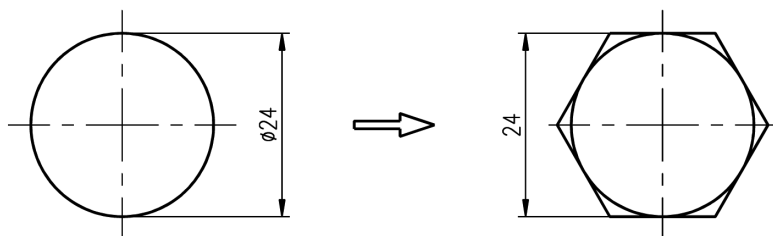
Polygon opsaný kolem kružnice
