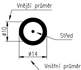
Obrázek č. 3.22: Konstrukce prstenu
