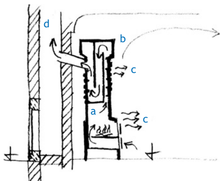
1.14 Účinnost kachlových kamen a – členitý povrch akumulace tepla, b – ohřívání, c – sálání, d – komin; účinnost 80%
